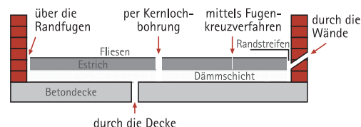
Verschiedene Varianten der Zuleitung trockener Luft unter den Estrich
