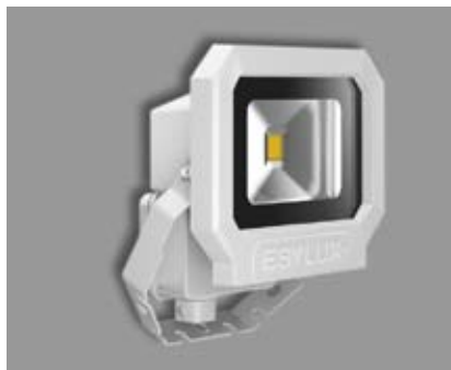
3225424.* Stahl verzinkt Silber Weiß EEK: A+, 2 x 2,5 W, LED-Modul tauschbar 3000 K, 360 lm H 270, A 115, L 170 € 67,70
