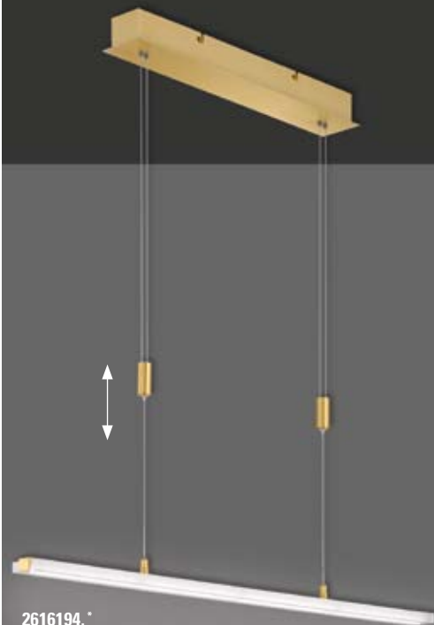
2616194.* Messing matt, Acrylglas Weiß matt EEK: A+ 25,2 W, LED 3000 K, 2520 lm L 840 dimmbar, Phasenabschnitt höhenverstellbar € 297,20
