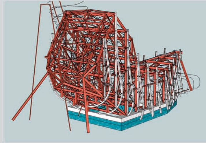
Holzkonstruktion für ein Piratenschiff im Heidepark Soltau (Statik und Ausführungszeichnungen)
