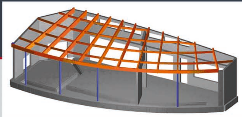
Anbau einer Schulmensa in Laatzen (Statik Beton-, Stahl- und Holzbau)
