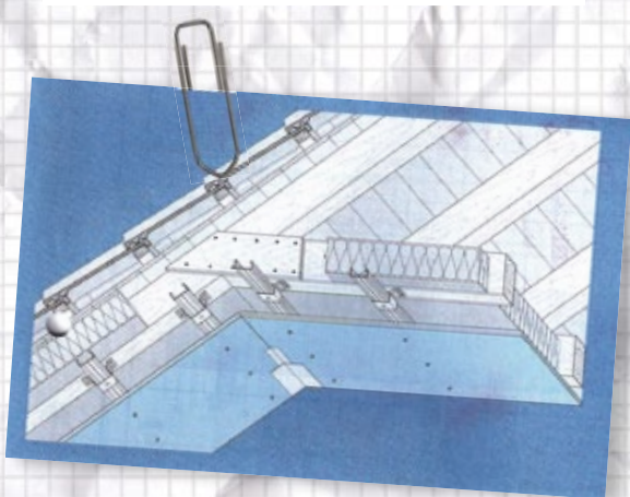
Dachgeschoss - Bekleidung
