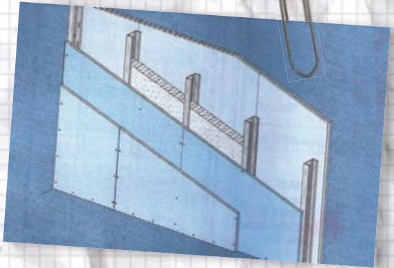
Metallständerwand
