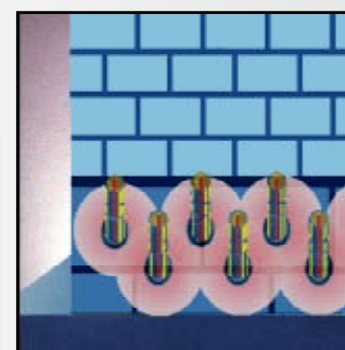
11. Schleierinjektion Decke, Wand, Boden Konstruktionsvergelung Geologische Verfestigung
